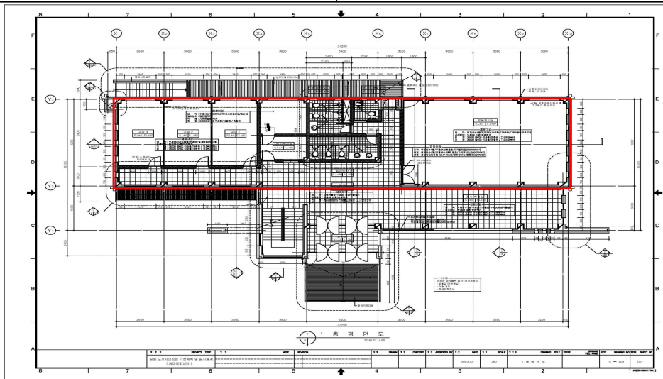
(평면도)
